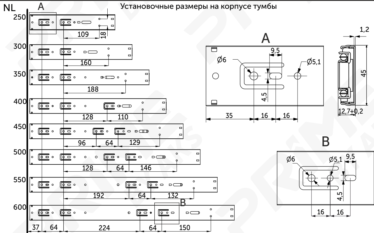
Установочные размеры на боковой стенке выдвижного ящика
